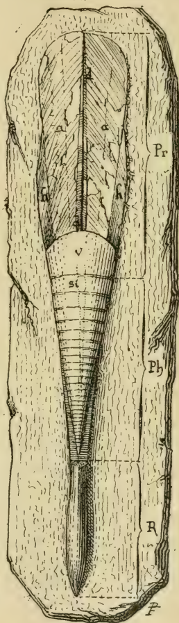
Fig. 363. — Belemnites .
